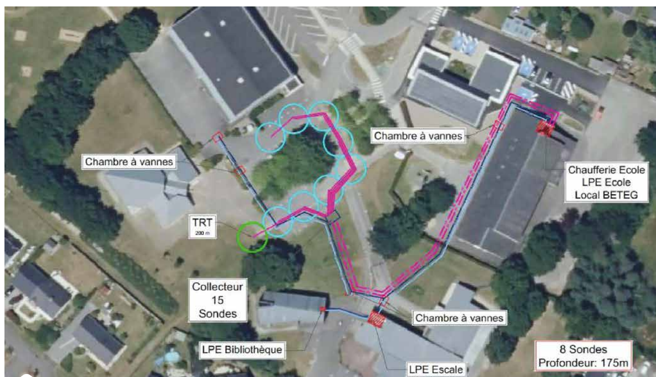
Schéma de principe des forages
